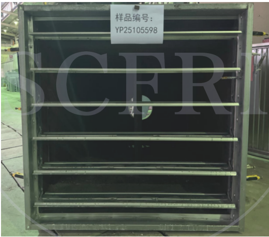
照片 1 耐火性能试验前试件情况
